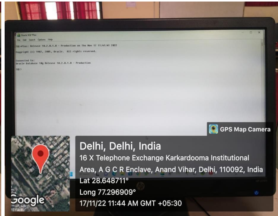
Oracle 9.0
